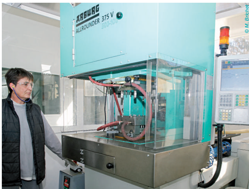
Presse à fermeture verticale dans une salle grise : surmoulage de matière plastique sur une pièce métallique.
